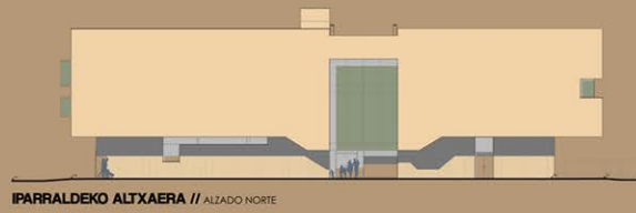
IPARRALDEKO ALTXAERA // ALZADO NORTE
